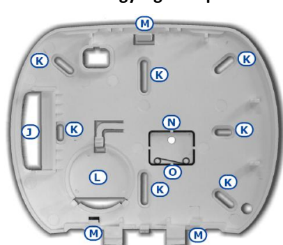
JOY kezelőegység hátlap
