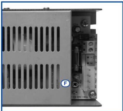
3A-es kapcsolóüzemű tápegység (SmartLiving 1050 és 1050L)
