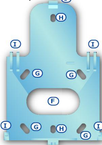
nCode/G kezelőegység szerelőlap
