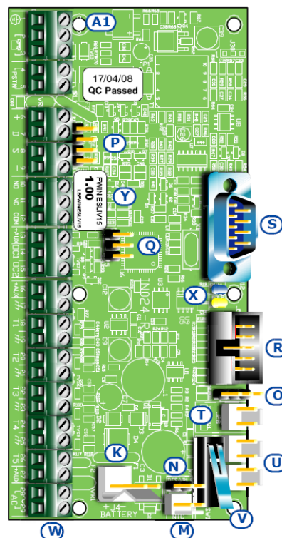
A SmartLiving515 központ alaplappja
