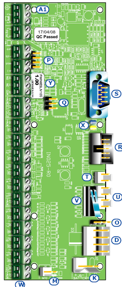
A SmartLiving 1050 / 1050L és 10100L központ alaplappja
