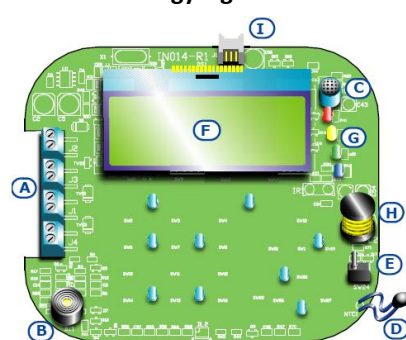
JOY kezelőegység PCB
